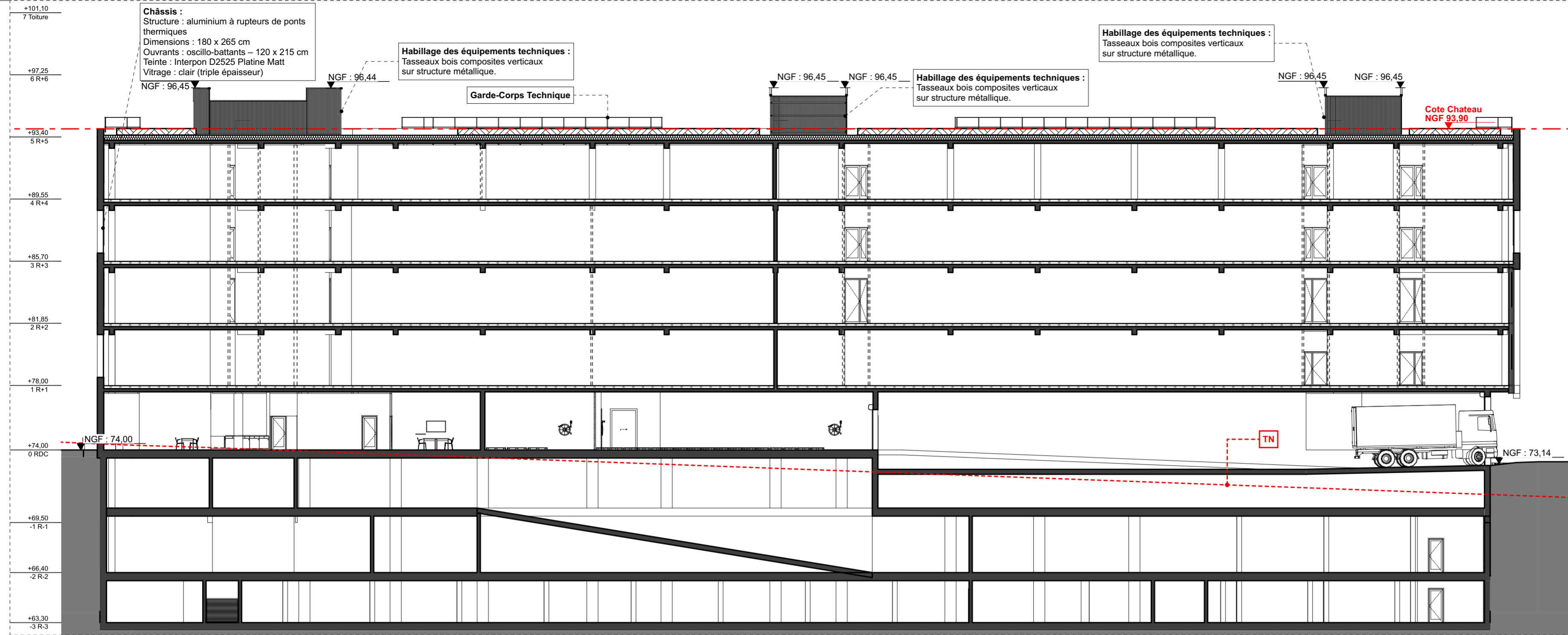
Coupe sur bâtiment D
